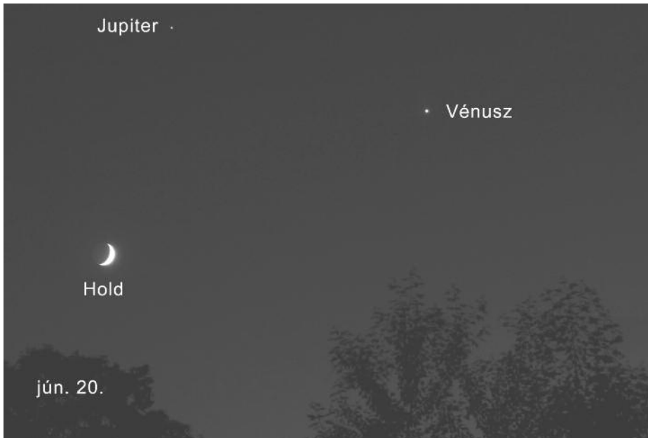
Vénusz–Jupiter (–Hold) együttállás 2015 június–júliusban
