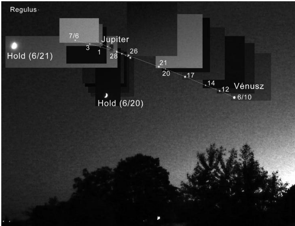
Vénusz–Jupiter (–Hold) együttállás 2015 június–júliusban
