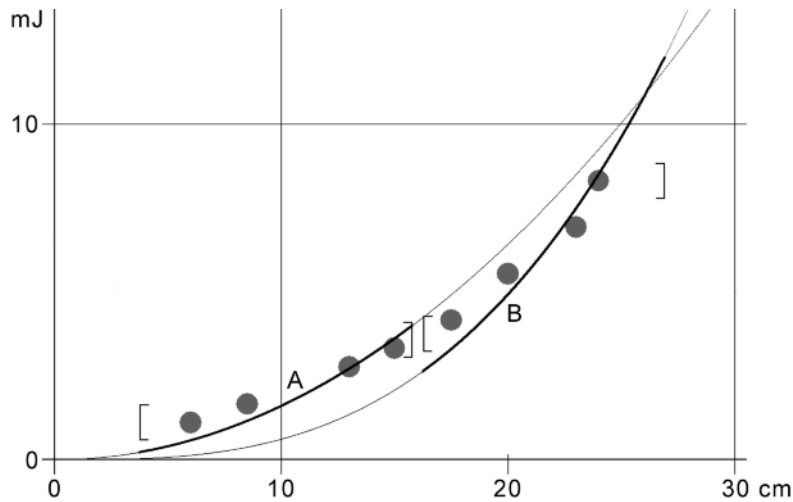
A teniszlabda-inga munka–amplitúdó függvénye
