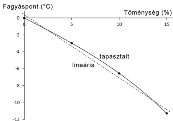
2. ábra A fagyáspont csökkenése a töménység függvényében
