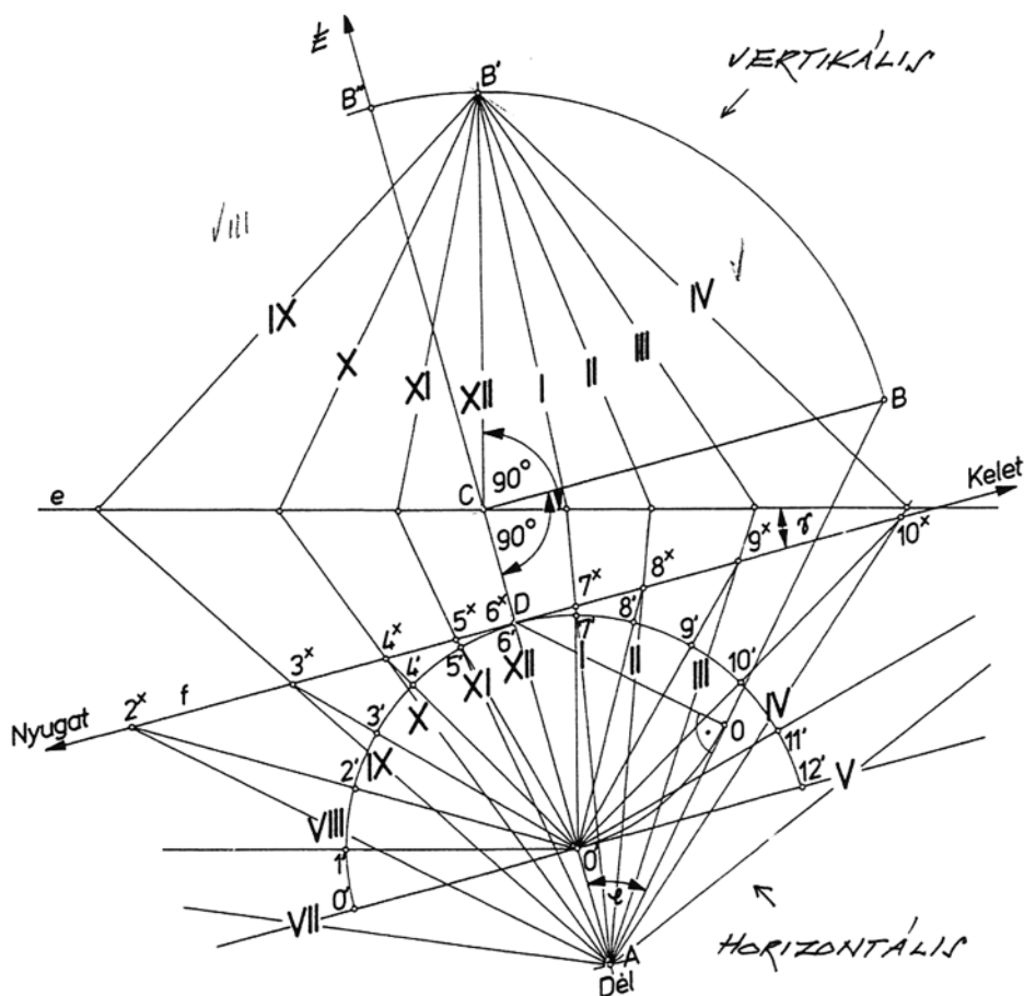
A napóra szerkesztési rajza
