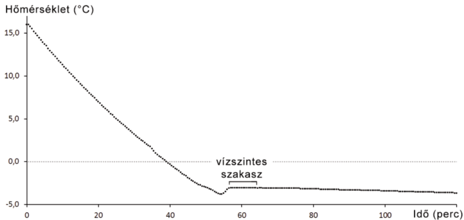
1. ábra Konyhasó 5%-os vizes oldatának hűlése és fagyása
