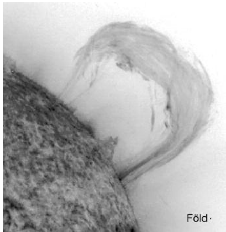
Óriási kitörés a Nap peremén (A SOHO űrszonda felvétele)
